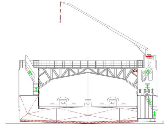
WR. 6 WIDOK W KIERUNKU DZIOBU
