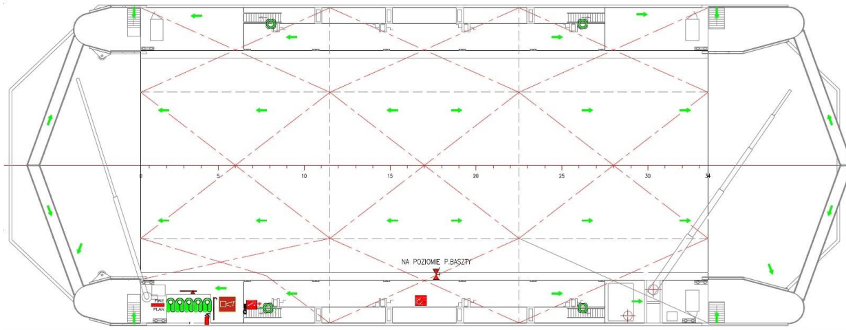
POKLAD ROBOCZY I POKLADY GÓRNE BASZT
